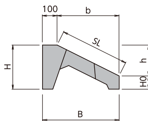
側面図
